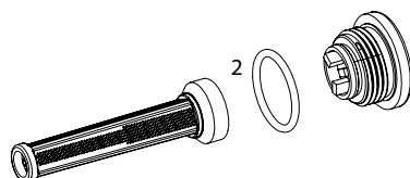
Ensemble pilote du tamis du filtre
